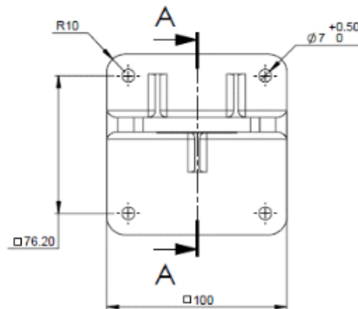
Рисунок 1: Основание наклонной крепежной базы - вид сзади
