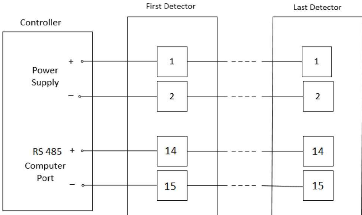
Рисунок 8: Сеть RS-485
